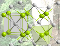
Fluoriet kristalstructuur
